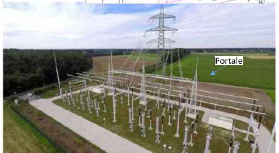
Beispiel KÜS für Wechsel Freileitung auf Erdkabel (hier ohne Drossel, Betriebsgebäude und Lager)
