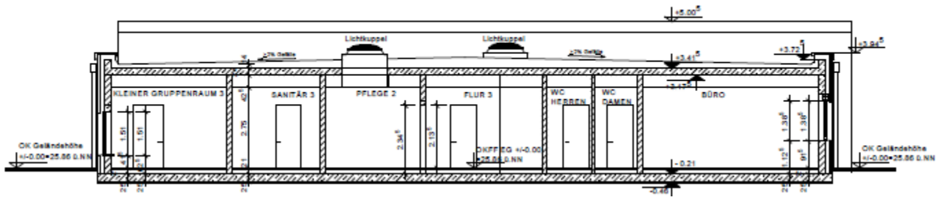
Schnitte
