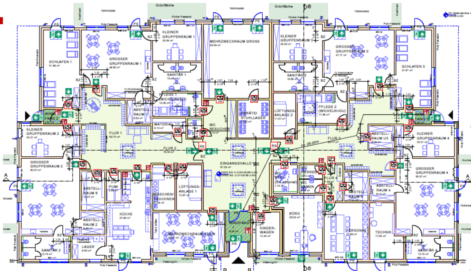
Grundriss
