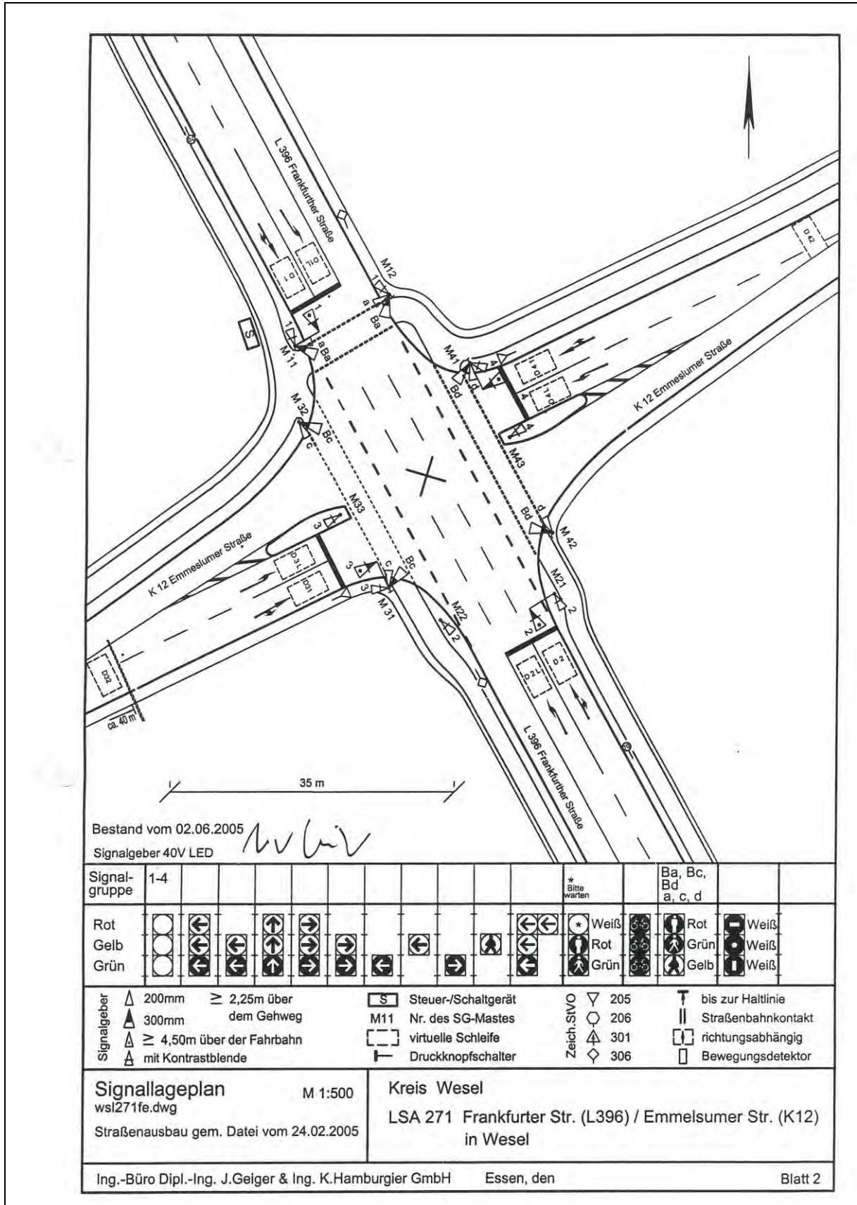
Abbildung 1: Signaltechnische Unterlagen zum Knotenpunkt Frankfurter Straße / Emmelsumer Straße - Signallageplan - (Quelle: Landesbetrieb Straßenbau NRW, Regionalniederlassung Niederrhein)
