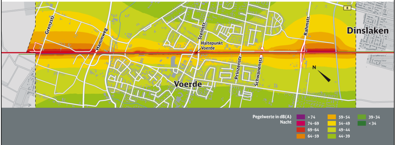
PFA 1.4 – Lärmpegel Prognose 2025 mit Schallschutz
