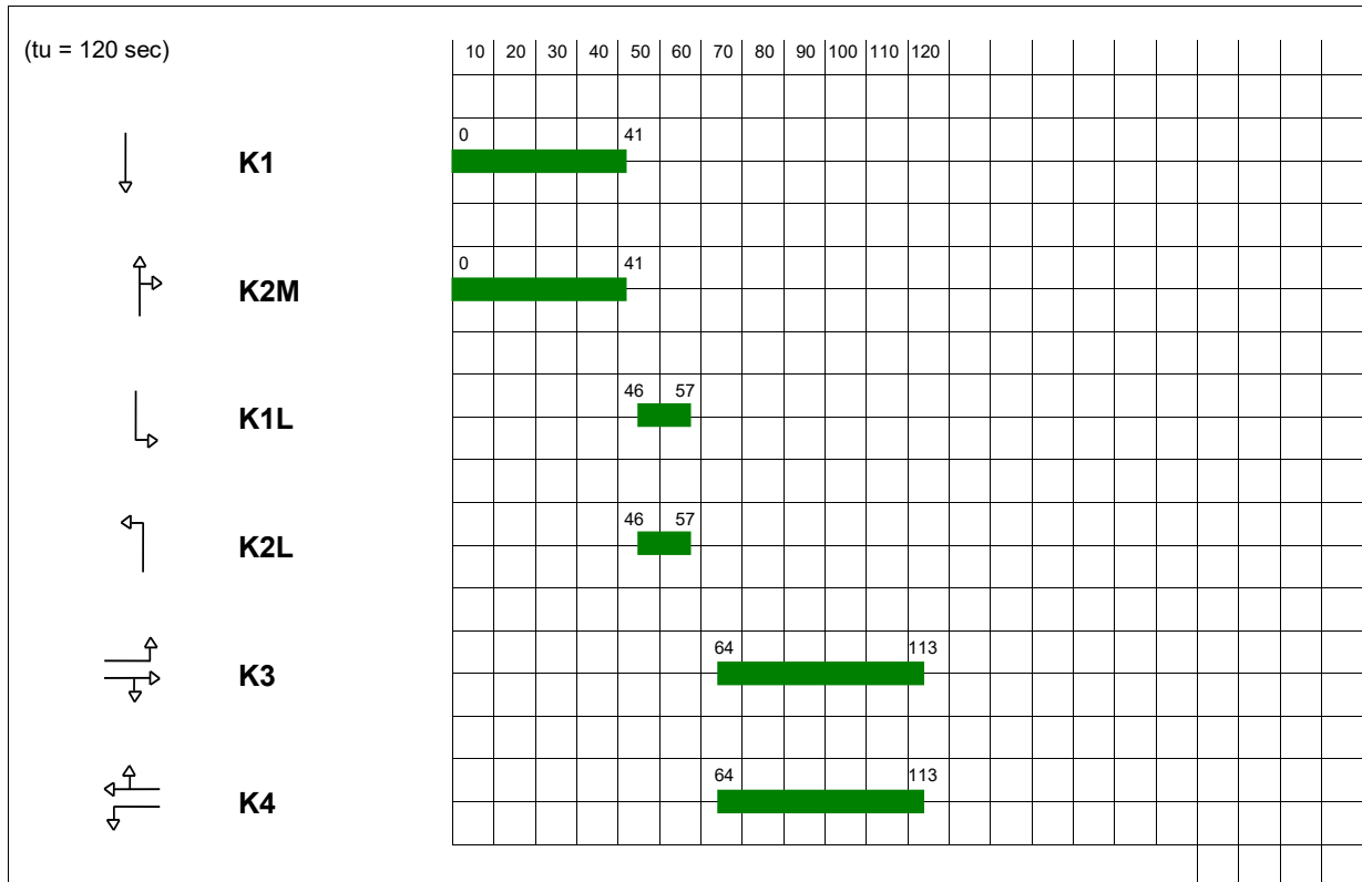
Abbildung 19: Anpassung des Festzeitprogramms am Knotenpunkt Willy-Brandt-Straße / Emmelser Straße / Neue Hünxer Straße in der Morgen- und Nachmittagsspitze
