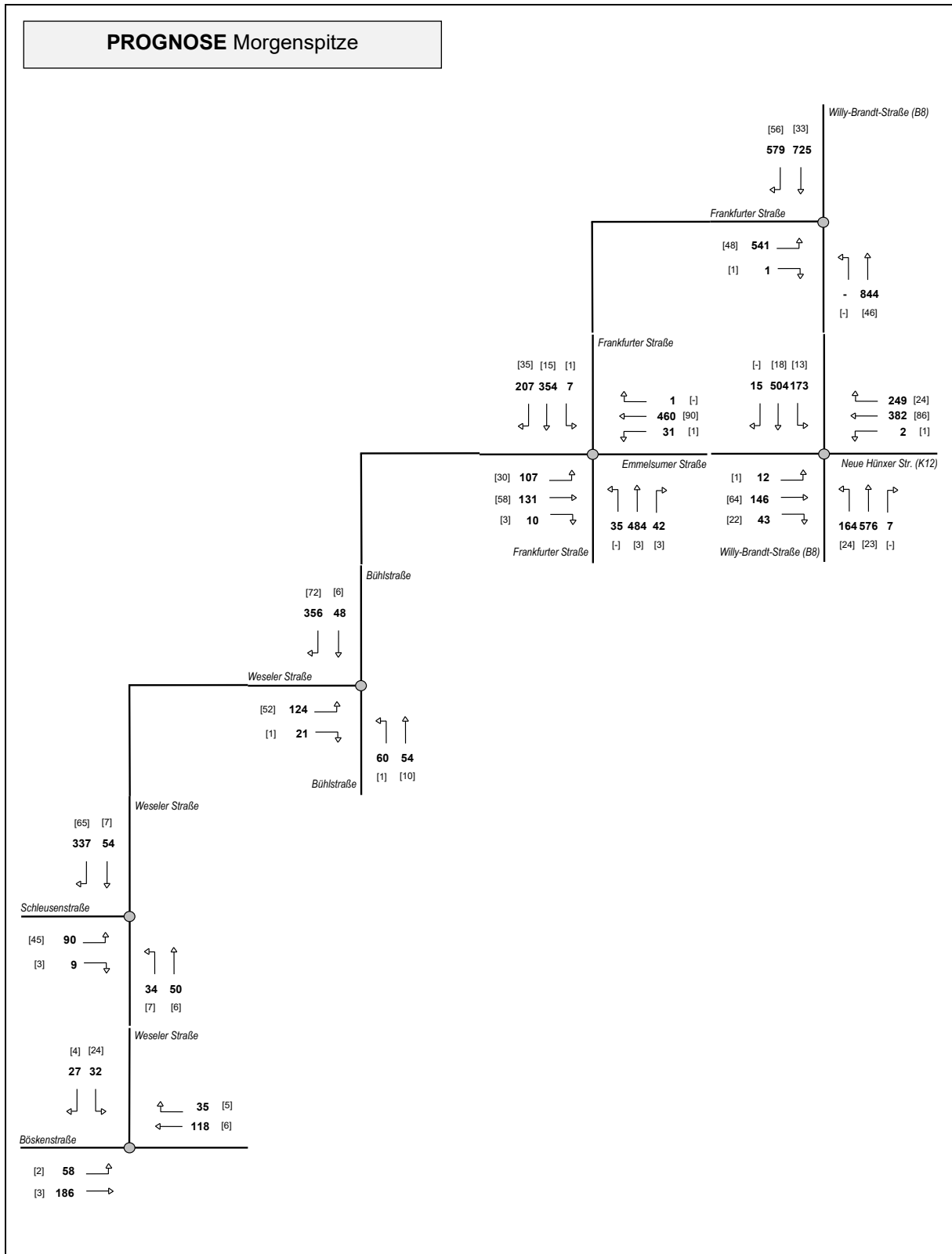
Abbildung 10: PROGNOSE-Verkehrsbelastungen [Kfz/h] an den umgebenden Knotenpunkten in der Morgenspitzenstunde (in Klammern: Anzahl der Fahrzeuge im Schwerverkehr)
