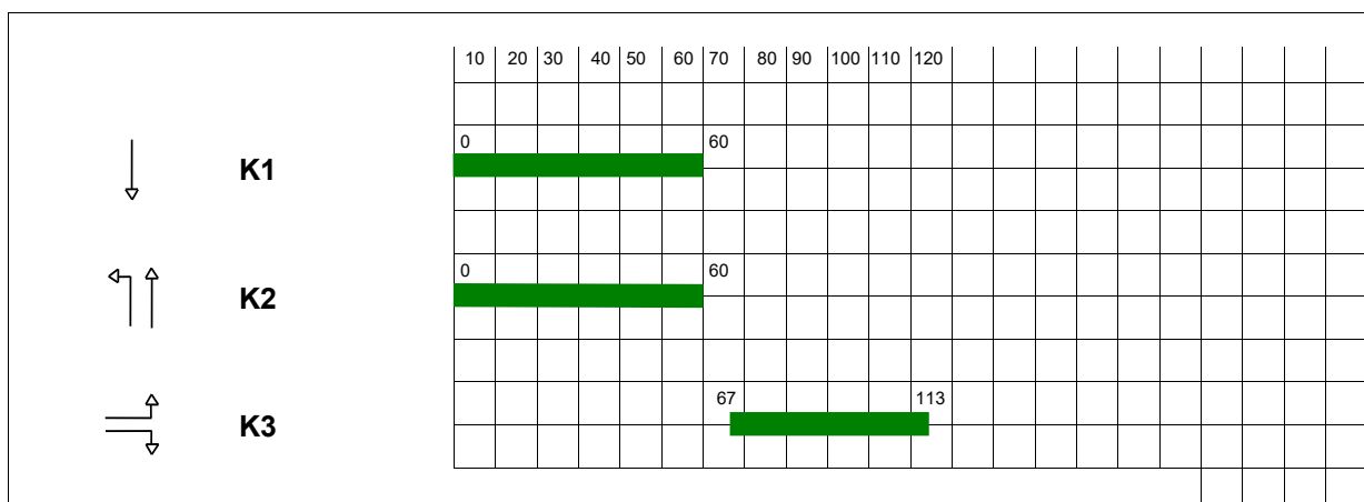
Abbildung 15: Anpassung des Festzeitprogramms am Knotenpunkt Willy-Brandt-Straße / Frankfurter Straße in der Morgen- und Nachmittagspitze
